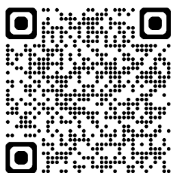
suvat
